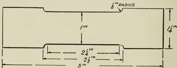
FIG. 201.—Tensile Strength Specimen.
